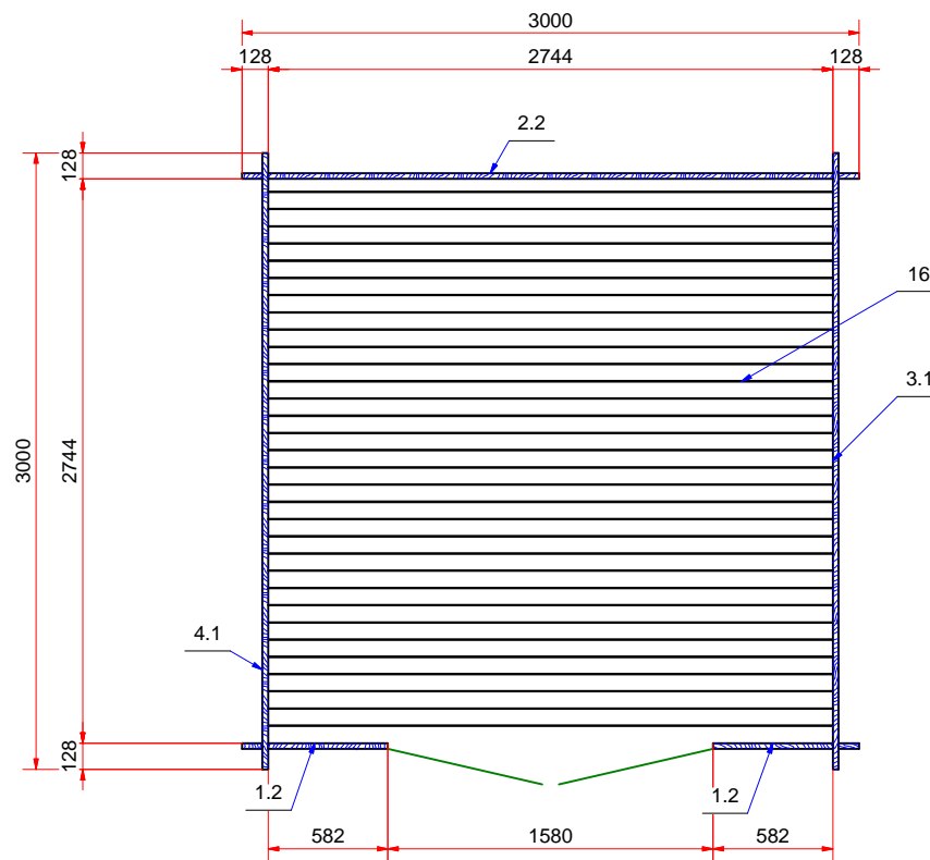
План дома (house plan)
