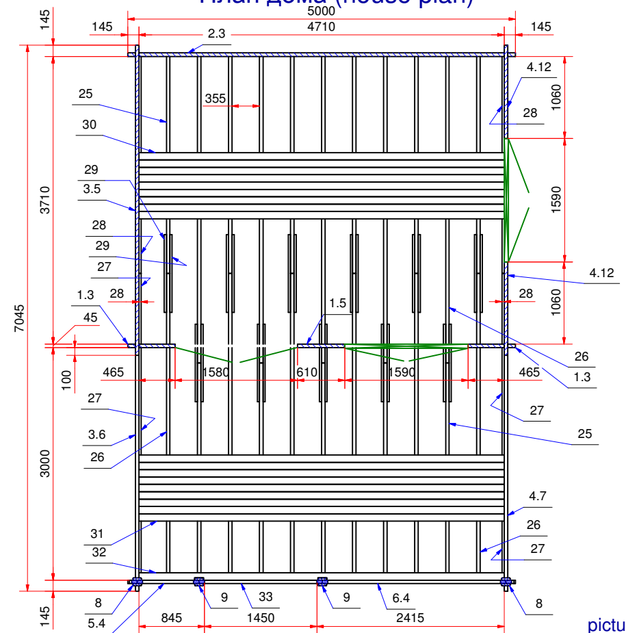
План дома (house plan)
